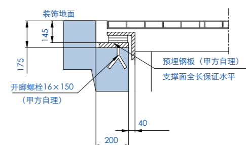
带防震橡胶垫或TEFLON滑垫支撑图
