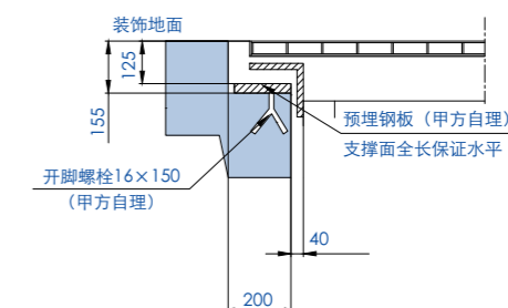
标准支撑图
