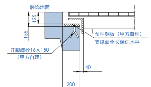
标准支撑图
