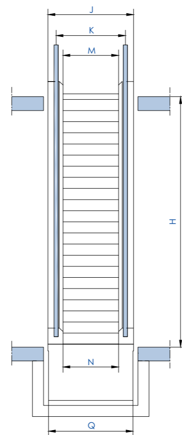
净通道区域 (上下平层) J × 2500mm 或 J × 2000mm
