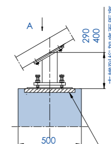
预埋钢板 (甲方自理) 30 × 400 × (400)
